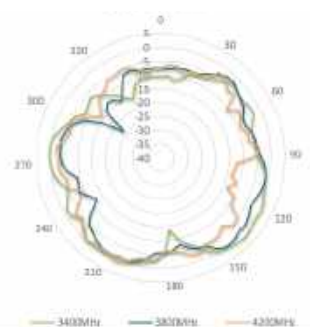
3400-4200 MHz
