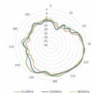
5150-5850 MHz
