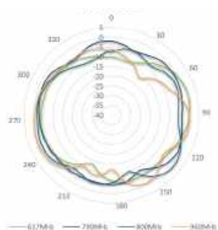
617-960 MHz
